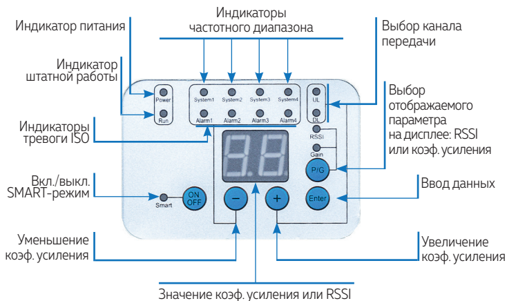
Рисунок 5 – элементы панели управления усилителя мощности сигнала
